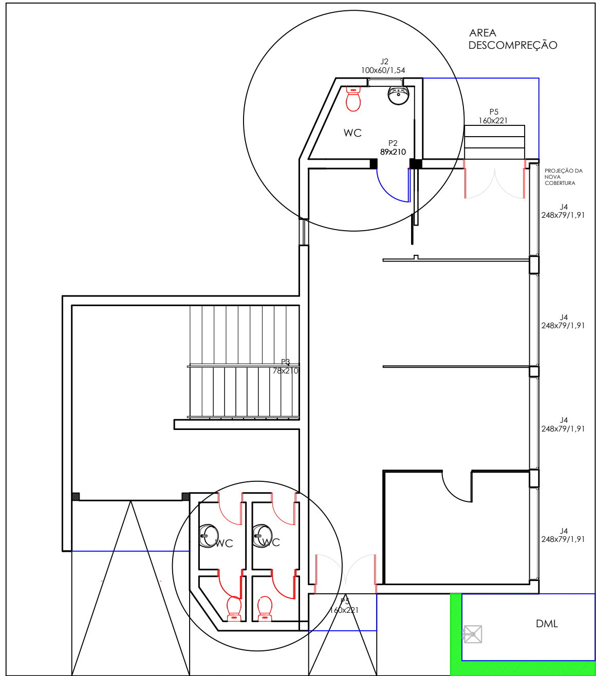
PONTOS DE ILUMINAÇÃO
