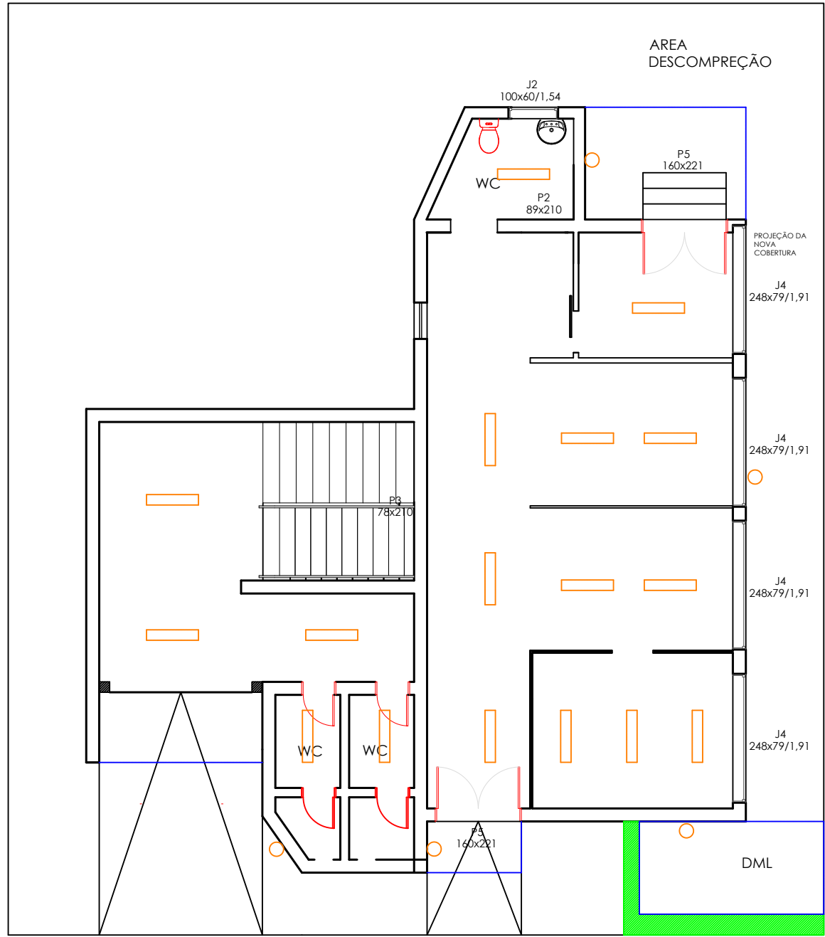
PONTO DE ILUMINAÇÃO PAVIMENTO SUPERIOR
