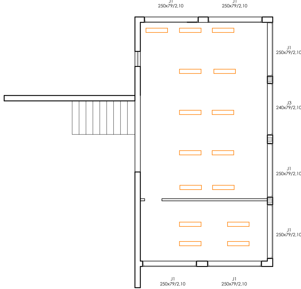
PONTO DE ILUMINAÇÃO PAVIMENTO TÉRREO
