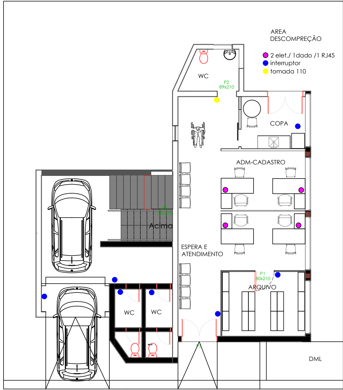
PONTO DE ELETRICA
