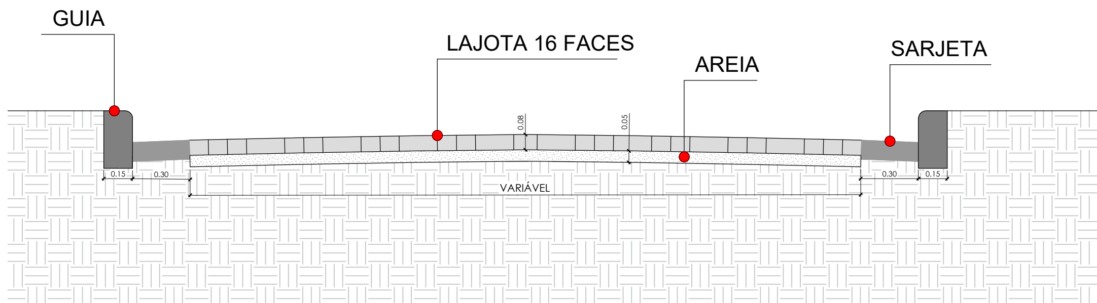
CORTE A - TRECHO COM REGULARIZAÇÃO ESCALA: 1:20
