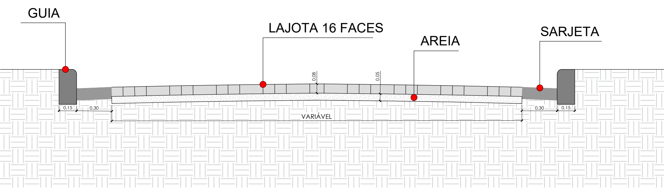
CORTE A - TRECHO COM REGULARIZAÇÃO ESCALA: 1:20
