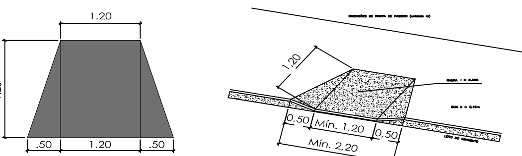
planta (03 pçs.) PREFEITURA MUNICIPAL SÃO BENTO DO SAPUCAÍ SP
