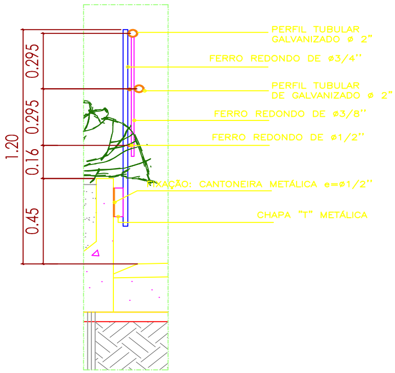
CORTE
