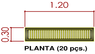
PLANTA / DET. GRELHA METÁLICA
