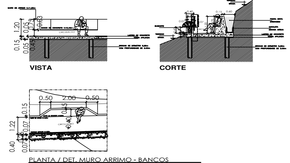
PLANTA / DET. MURO ARRIMO - BANCOS PREFEITURA MUNICIPAL SÃO BENTO DO SAPUCAÍ SP
