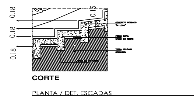
PLANTA / DET. ESCADAS PREFEITURA MUNICIPAL SÃO BENTO DO SAPUCAÍ SP
