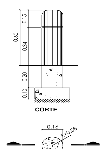
PLANTA / DET. BOLETES DE PROTEÇÃO DE CONCRETO PREFEITURA MUNICIPAL SÃO BENTO DO SAPUCAÍ SP
