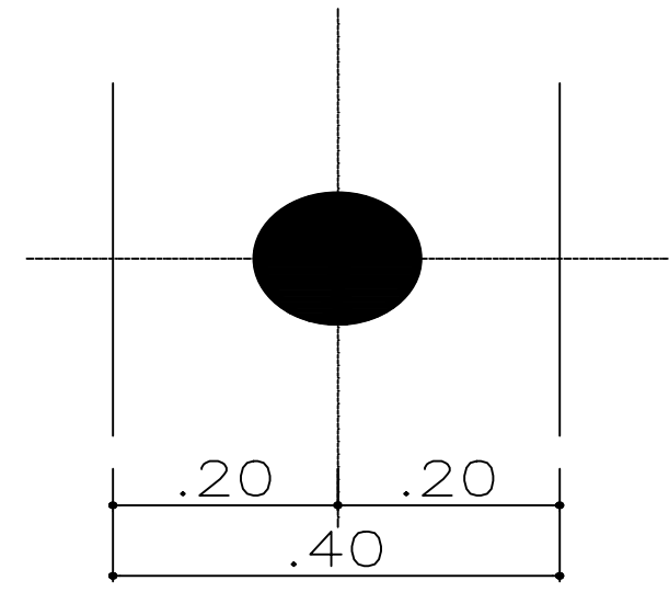
PLANTA (161 unidades)
