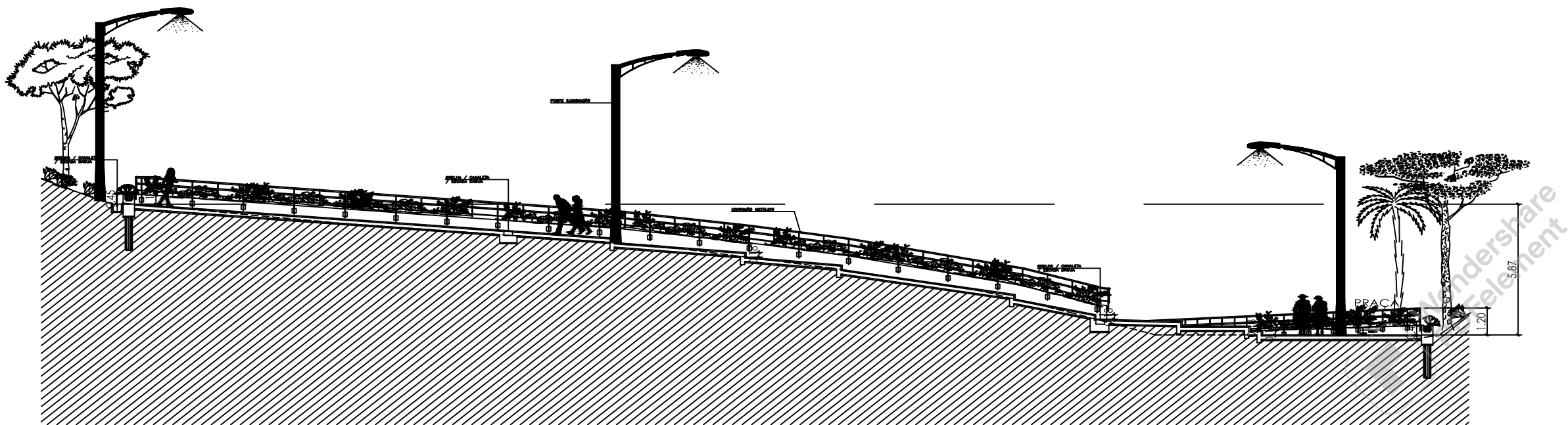
CORTE BB PREFEITURA MUNICIPAL SÃO BENTO DO SAPUCAÍ SP — escala 1:125
