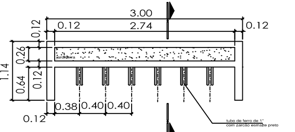
DETALHE BIBICLETARIO PREFEITURA MUNICIPAL SÃO BENTO DO SAPUCAÍ SP
