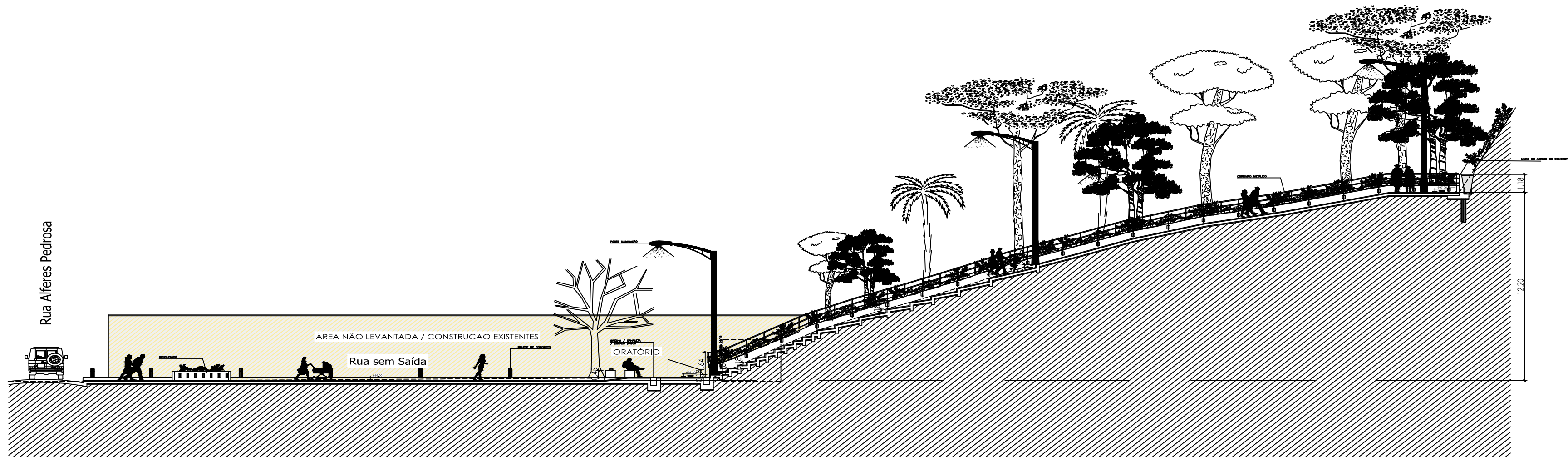
CORTE AA PREFEITURA MUNICIPAL SÃO BENTO DO SAPUCAÍ SP — escala 1:125
