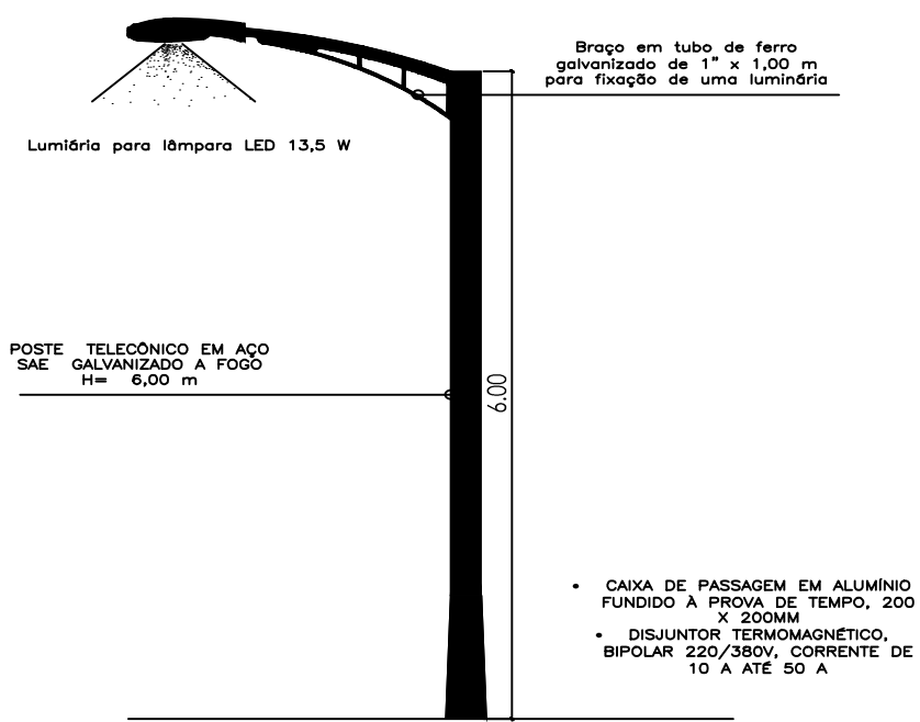
VISTA (23 pcs.)
