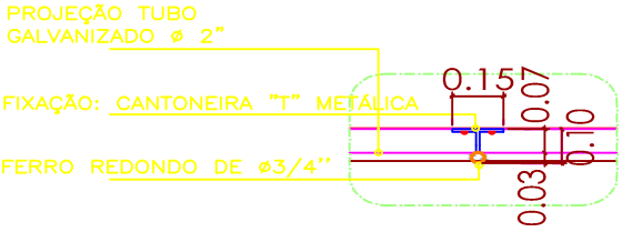
PLANTA / DET. GENÉRICO FIXAÇÃO
