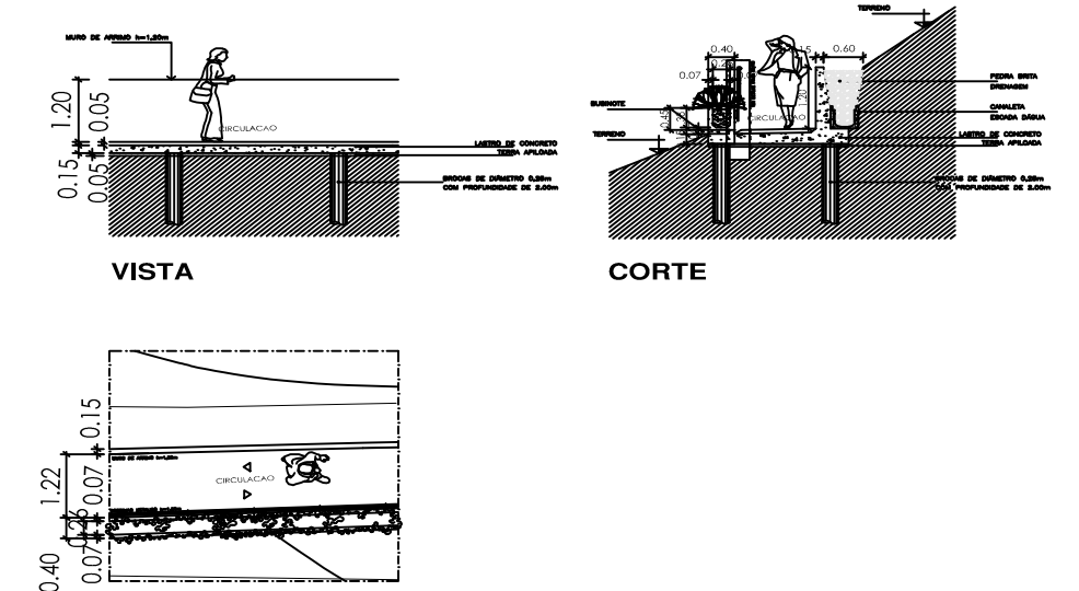
PLANTA / DET. MURO ARRIMO PREFEITURA MUNICIPAL SÃO BENTO DO SAPUCAÍ SP
