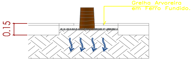
CORTE
